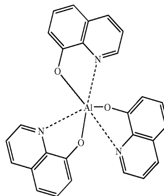
Alq3
